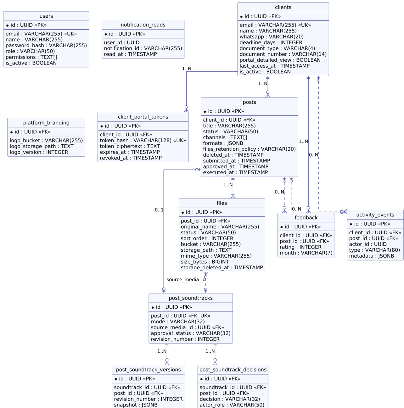
Figura 1: Diagrama Entidade-Relacionamento
